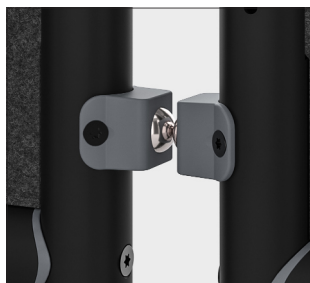
Enchaînement des cloisons entre elles
