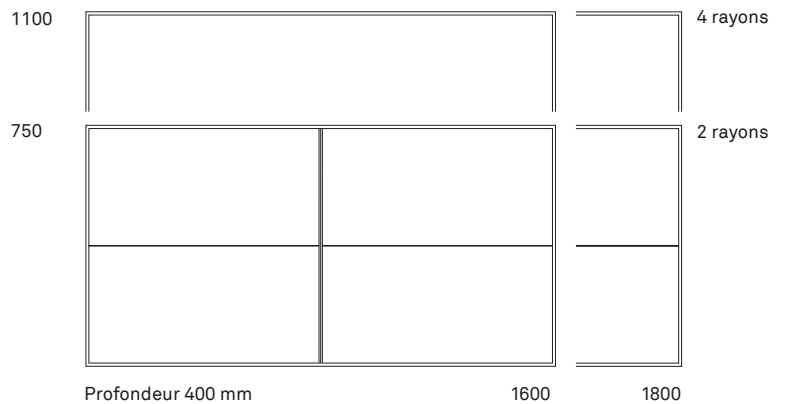
Profondeur 400 mm
