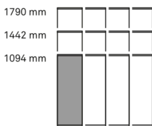
Housing Alloggiamento
